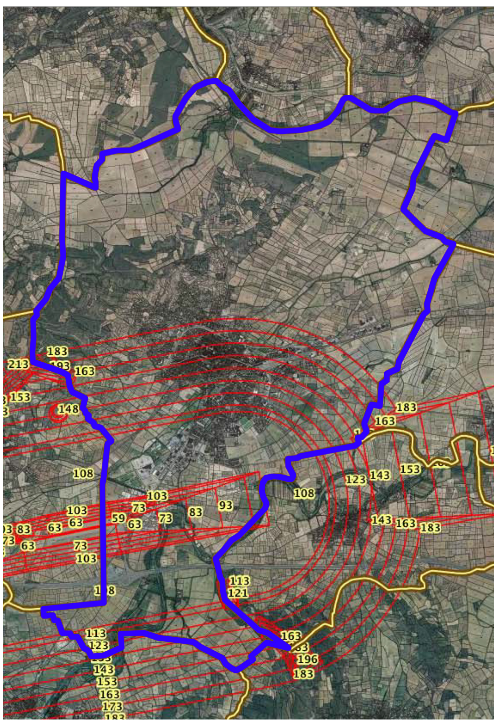
T5 - Servitudes aéronautiques Servitudes de dégagement (aérodromes civils et militaires) Code de l'aviation civile
